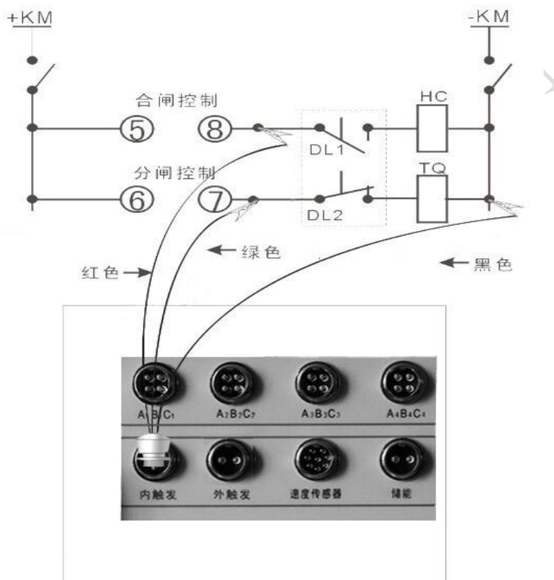
内触发控制接线示意图
