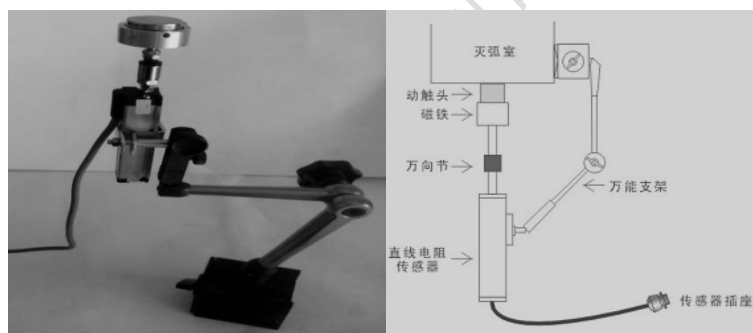
0.1mm 电子尺和万向节
