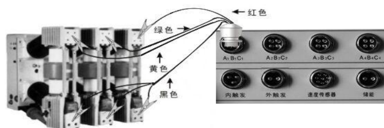
断口接线图（三断口）
