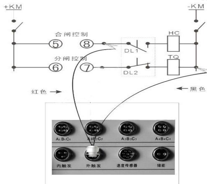
合闸外触发接线示意图
