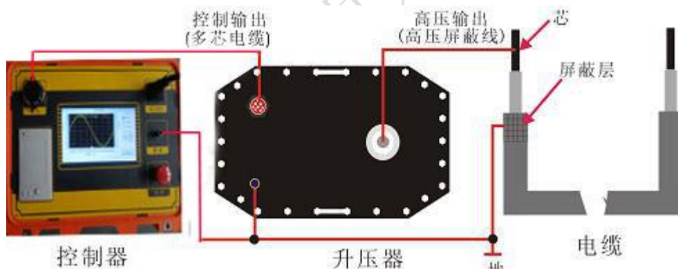
图8 单相电缆耐压测试接线图
